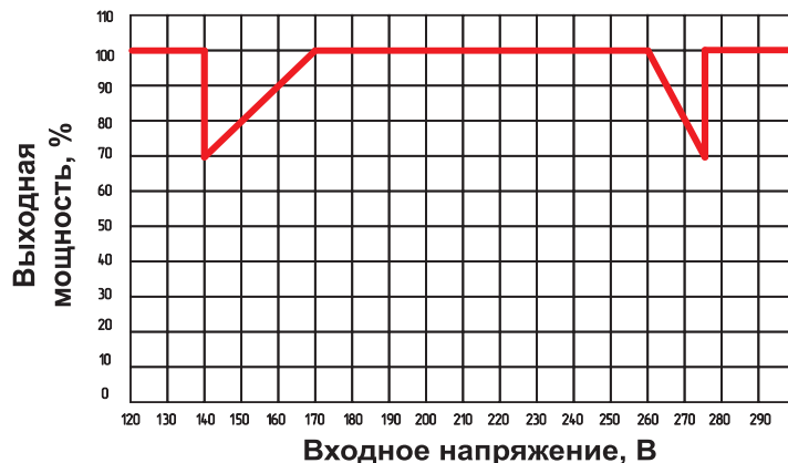
Рис.4 Максимальная мощность нагрузки в зависимости от напряжения сети.
